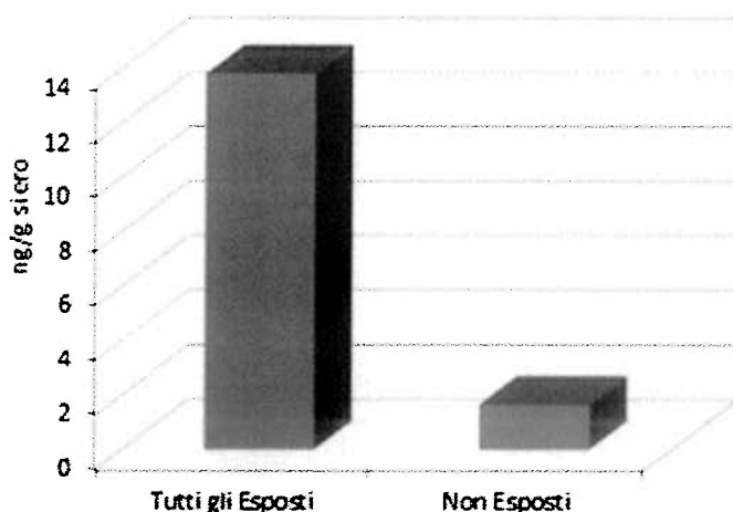
Concentrazioni (mediane) di PFOA nel siero di tutti gli Esposti e dei Non Esposti
